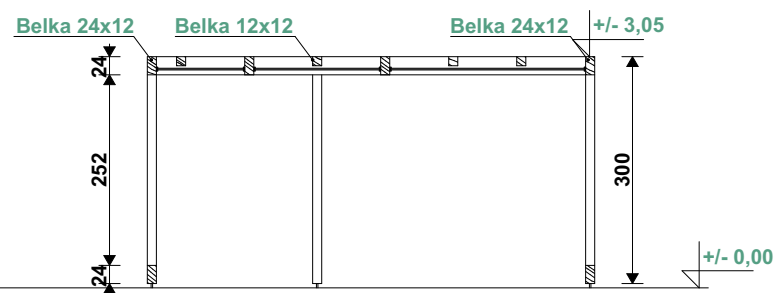
PRZEKRÓJ A-A 1:100
