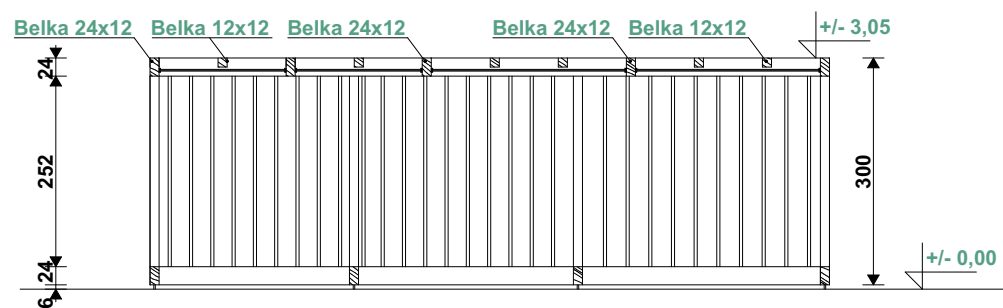
PRZEKRÓJ A-A 1:100
