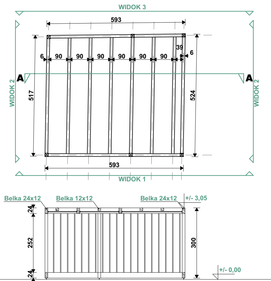
PRZEKRÓJ A-A 1:100
