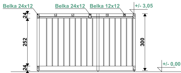
PRZEKRÓJ A-A 1:100
