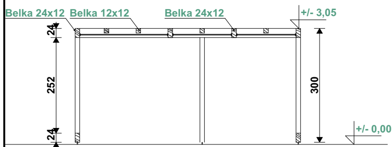
PRZEKRÓJ A-A 1:100
