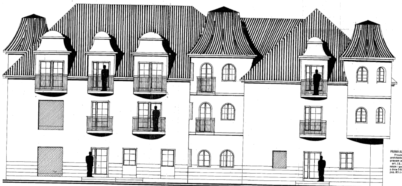
ELEWACJA WSCHODNIA
